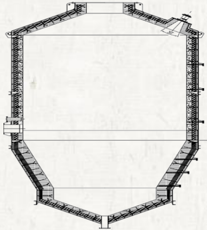
유동식 소각로
