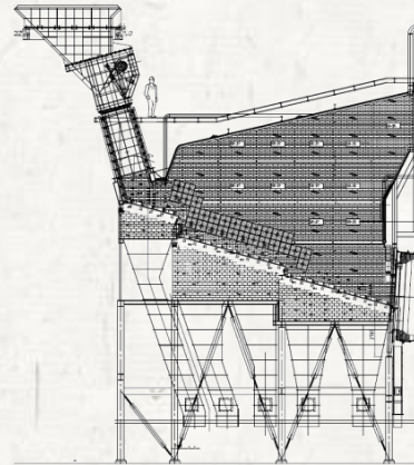
스토카식 소각로
